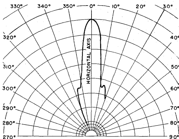
Fig. 12—Vertical diagram.
