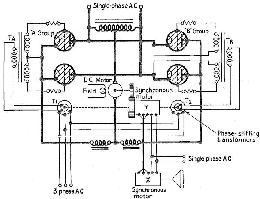
Fig. 41—Torque amplifier.
