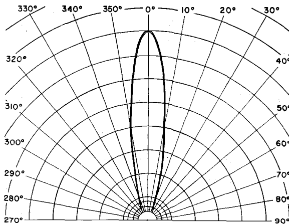
Fig. 11—Horizontal diagram.
