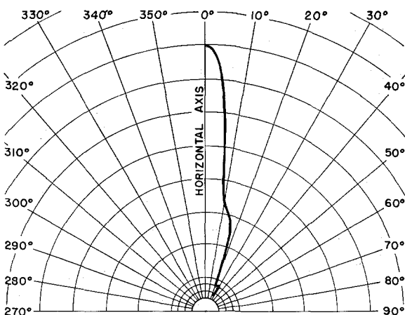
Fig. 13—Vertical diagram.
