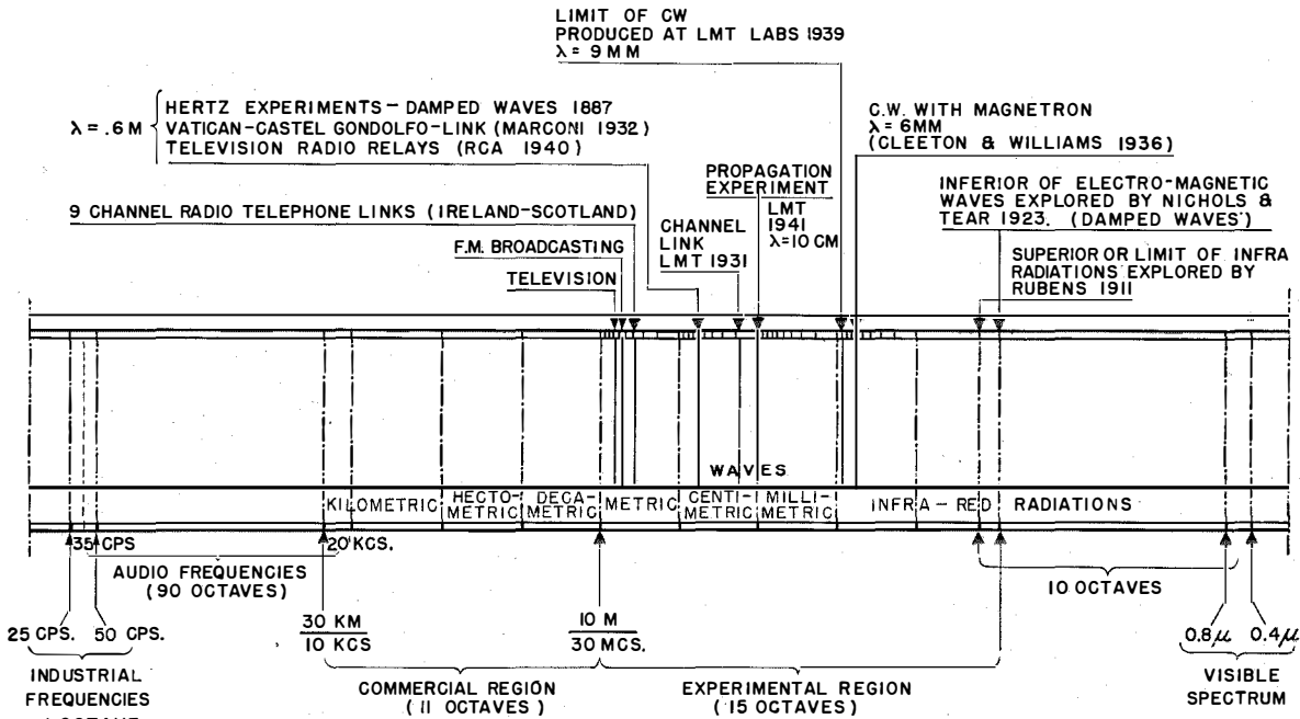
Fig. 1—Short-wave spectrum.
